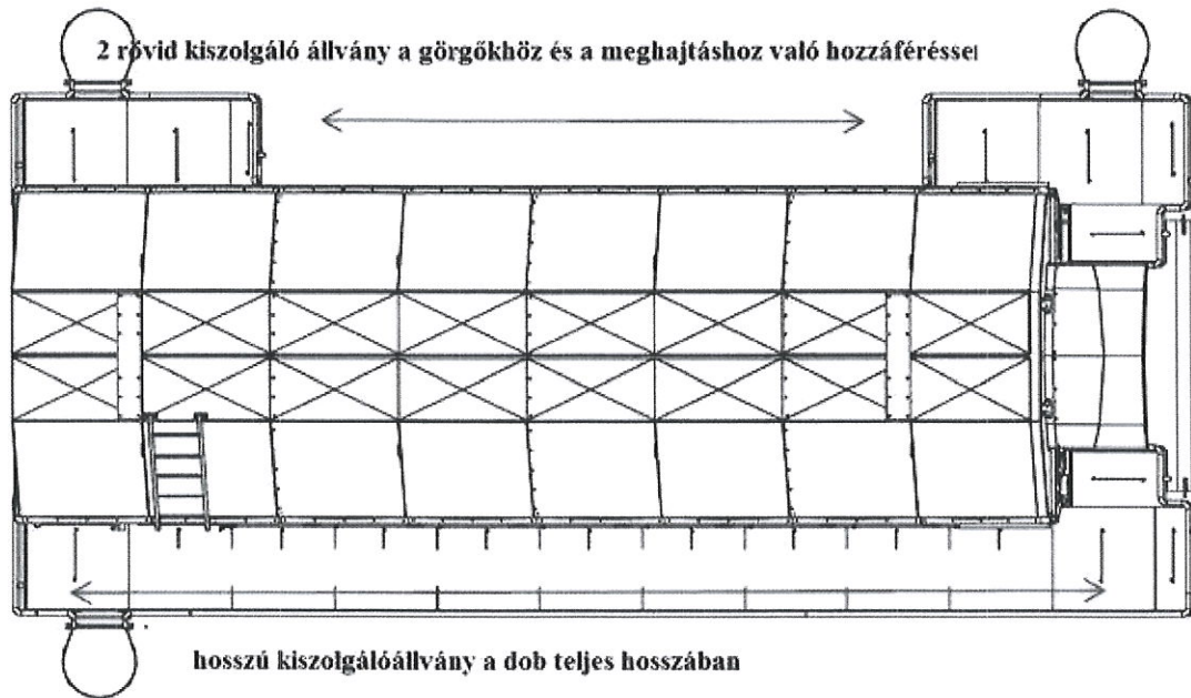
2 ábra: dobrosta felülnézetben, munkaállványokkal
